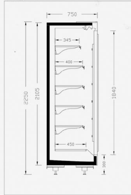
INVERNO 75-225
