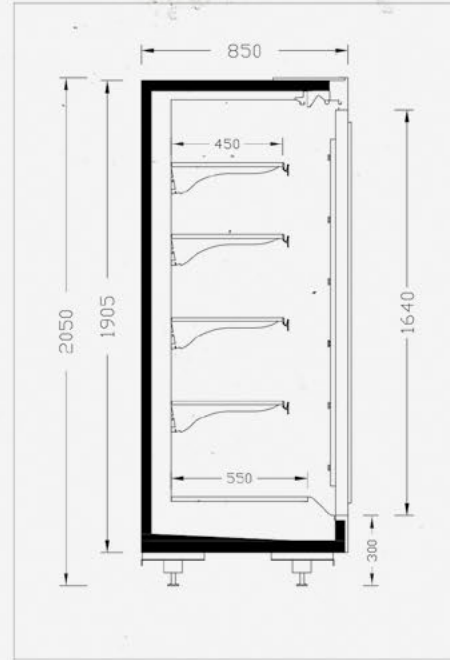
INVERNO 85-205
