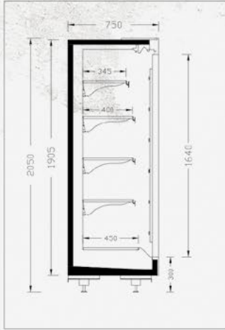
ELITE HD 75-205
