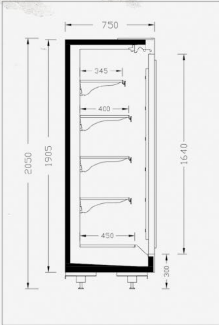
INVERNO 75-205
