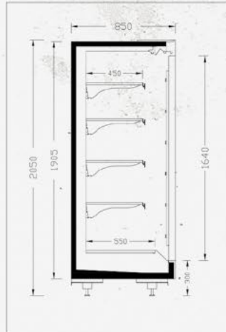
ELITE HD 85-205
