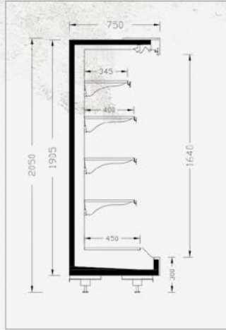
ELITE DD 75-205
