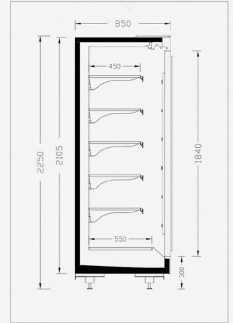
INVERNO 85-225
