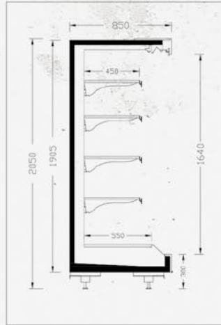
ELITE DD 85-205
