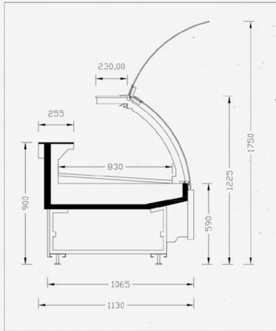
LATTERIA CG
