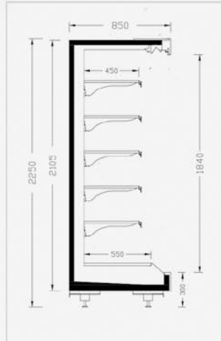
ELITE DD 85-225
