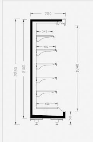
ELITE DD 75-225
